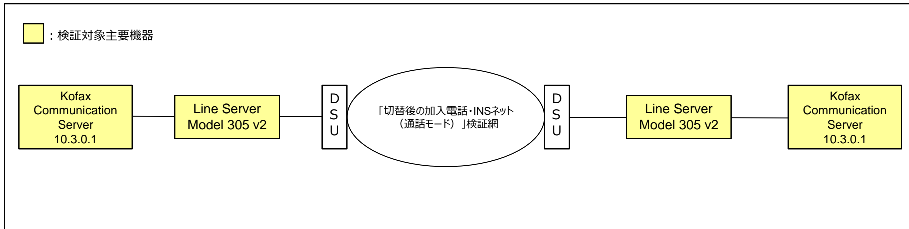
検証機器構成図
