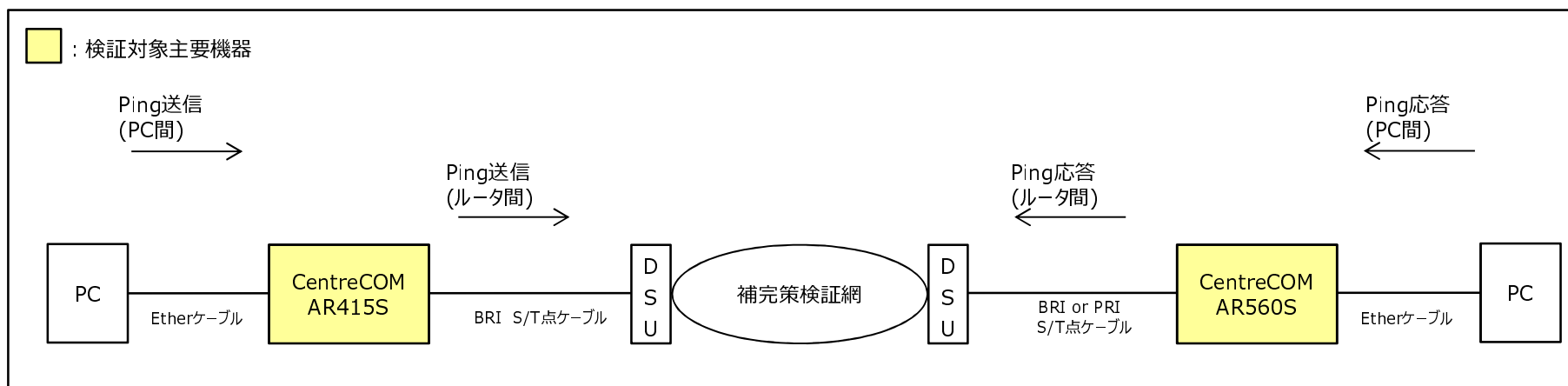
検証機器構成図
