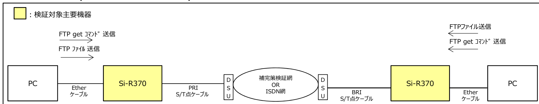
検証機器構成図2
