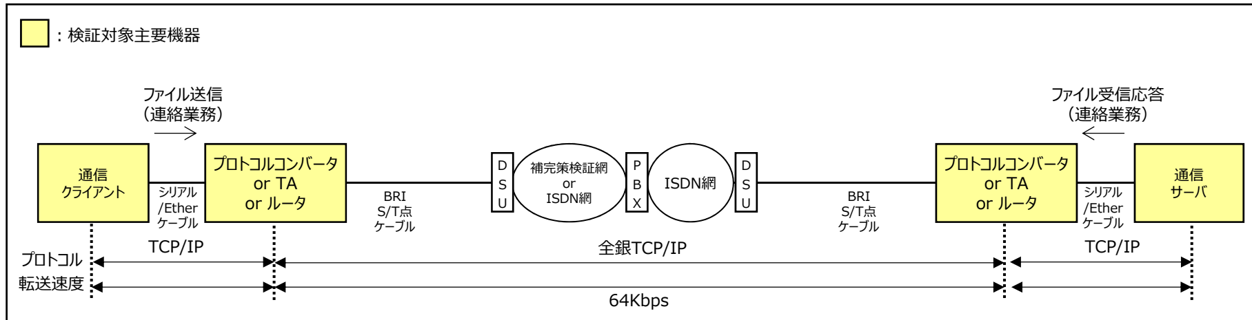
検証機器構成図4
