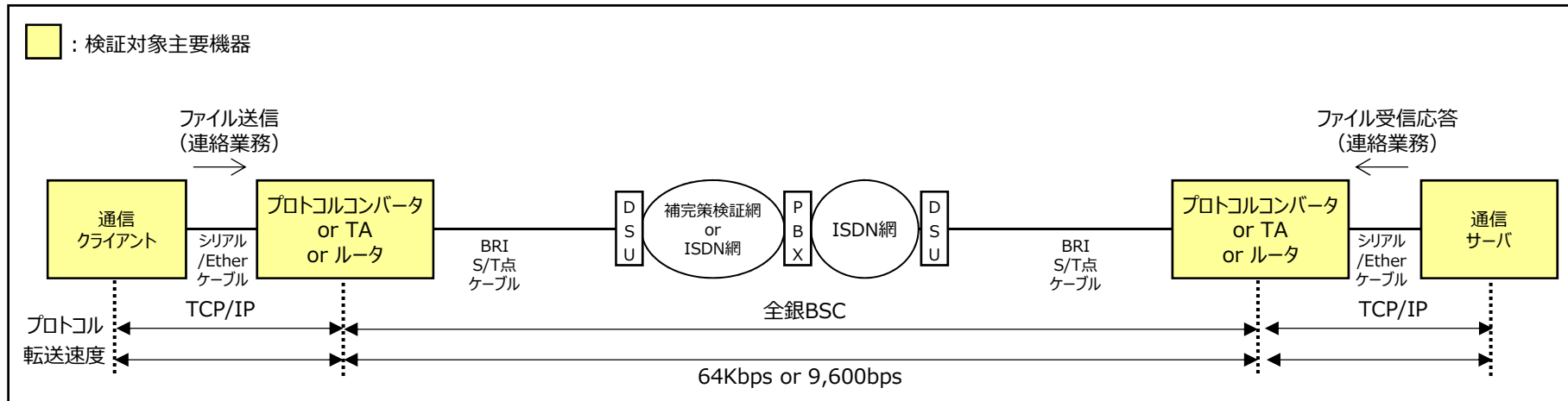
検証機器構成図2
