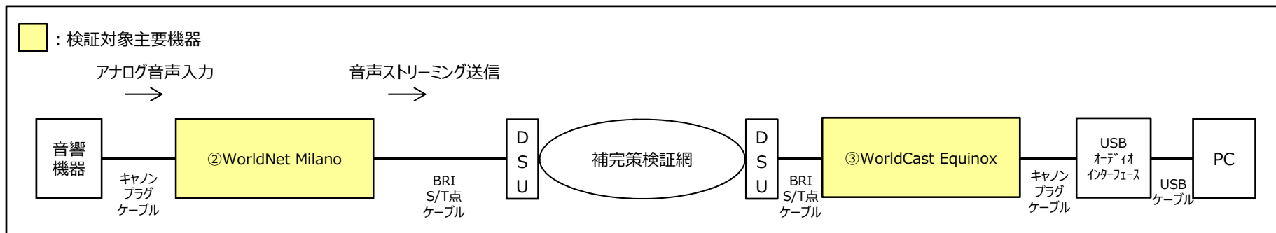
検証機器構成図 4
