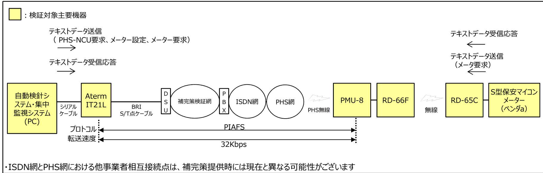
検証機器構成図2
