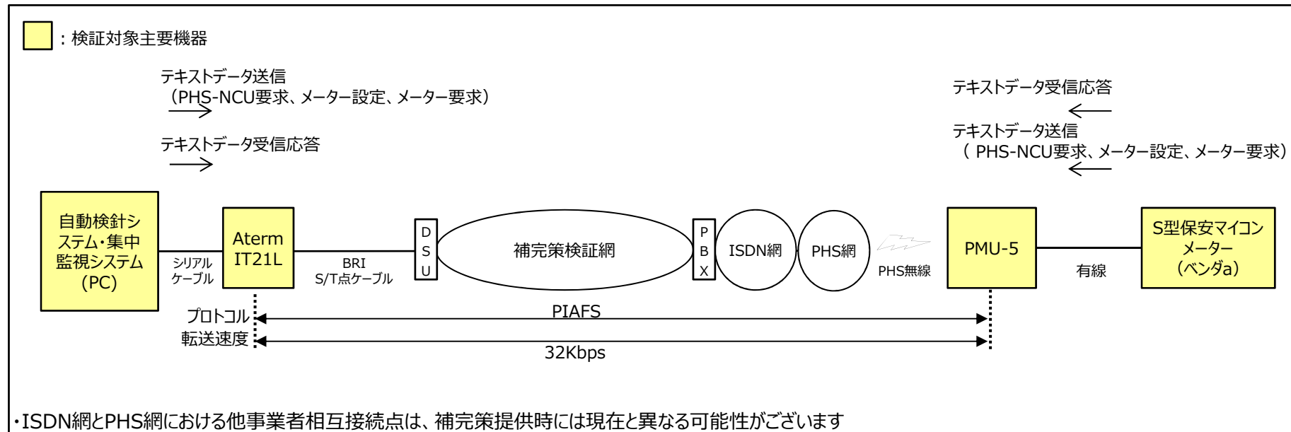
検証機器構成図1
