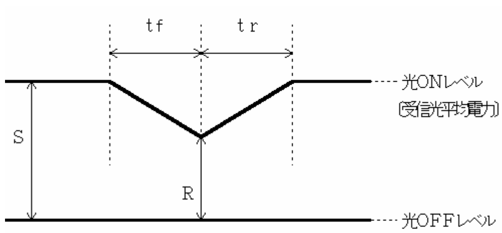
付図7 光レベル変動耐力測定波形
