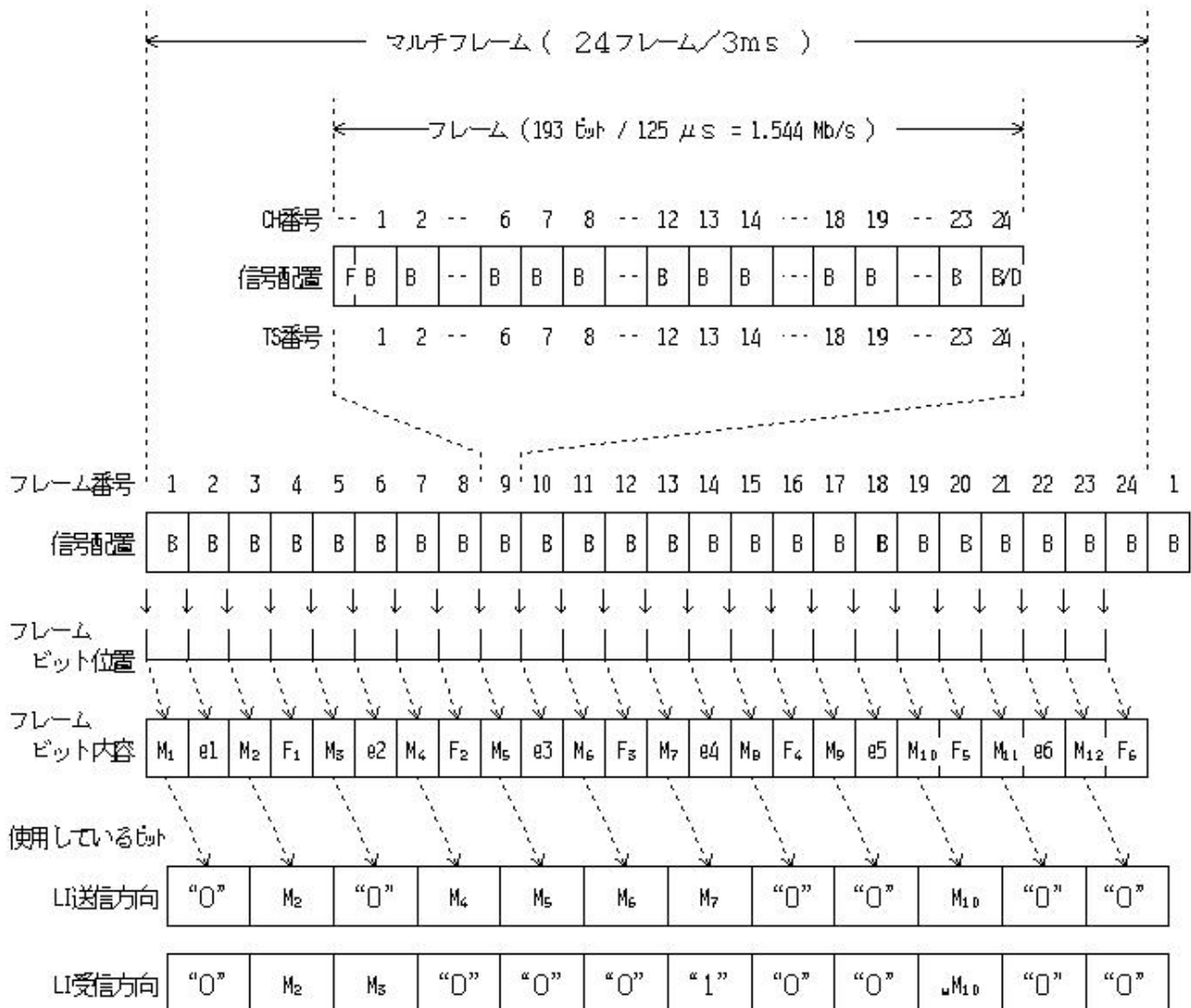
付図2 加入者線フレームフォーマット
