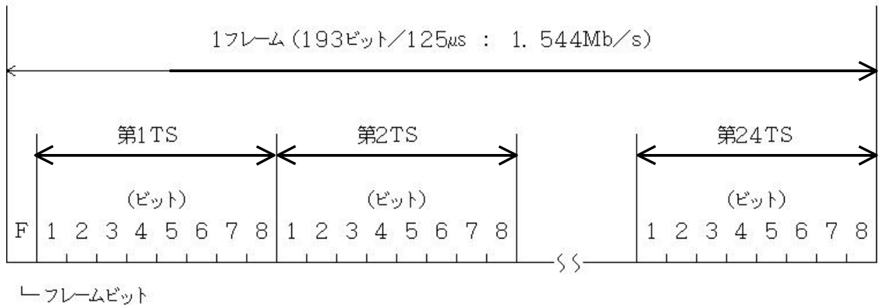
付図 1 1. 544 Mb/s フレーム構成
