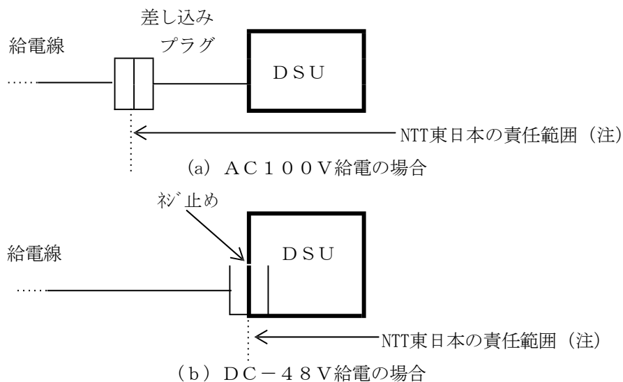
図 1. 4 施工・保守上の責任範囲（通信線）
