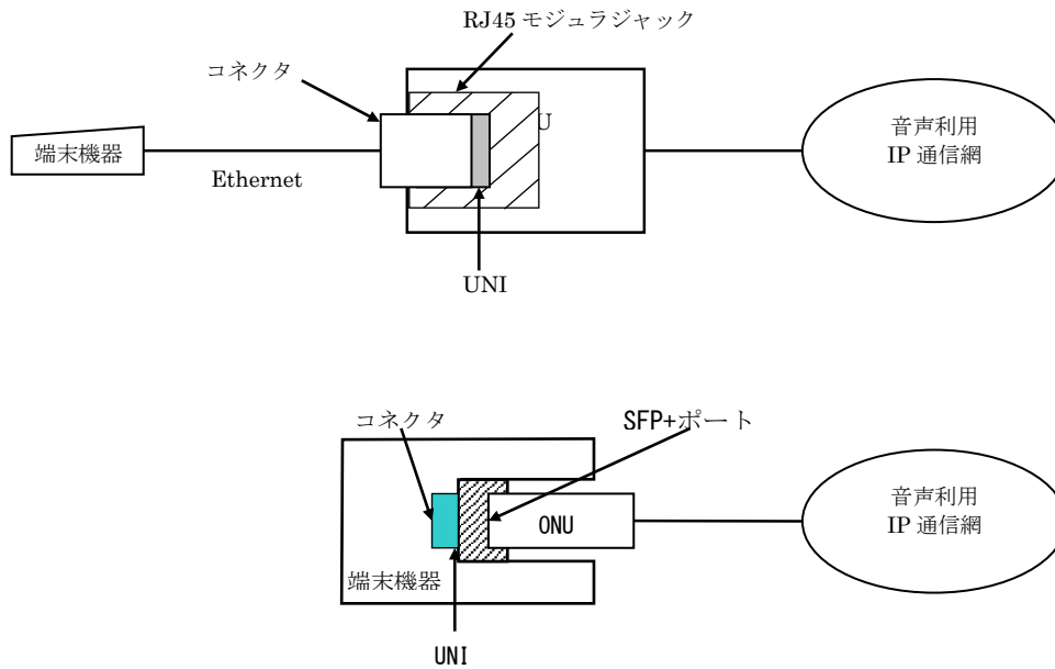
図 2-1：インタフェース規定点
