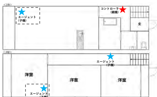
ケースC-1：（2階建て階段付近に親機）
